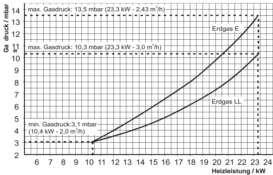
Abb. 5.9 Gas-Leistungsdiagramm Erdgas
