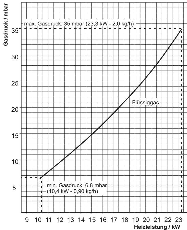
Abb. 5.10 Gas-Leistungsdiagramm Flüssiggas
