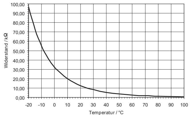
Abb. 4.12 Widerstandskurve
