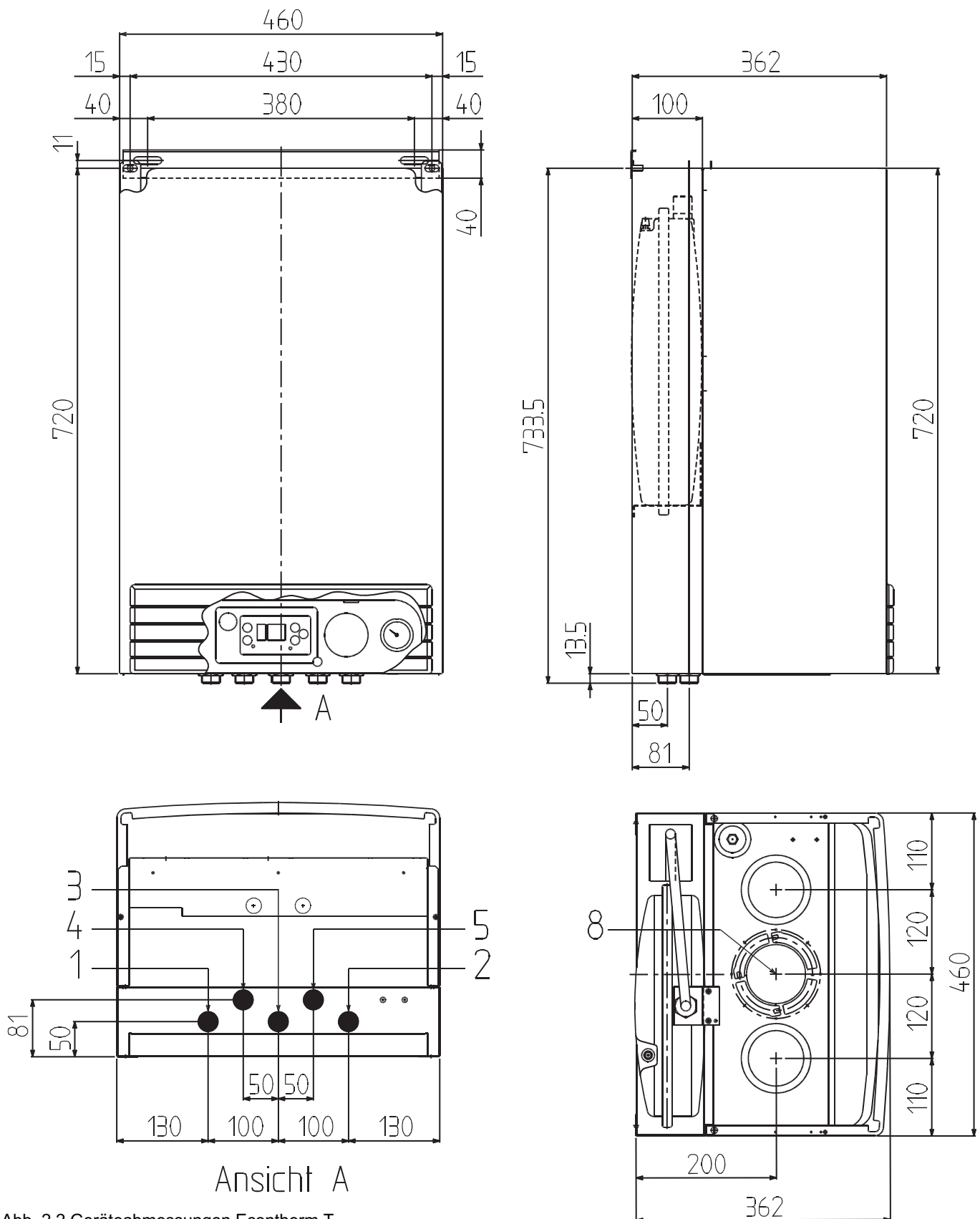
Abb. 2.2 Geräteabmessungen Econotherm T
